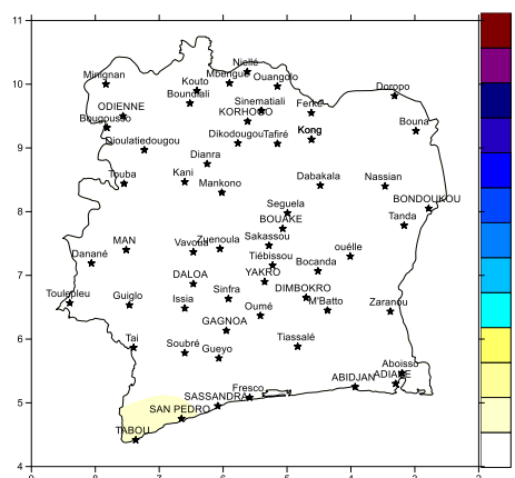
Fig1 : Pluviométrie totale (mm) du 11 au 20 Janvier 2020
