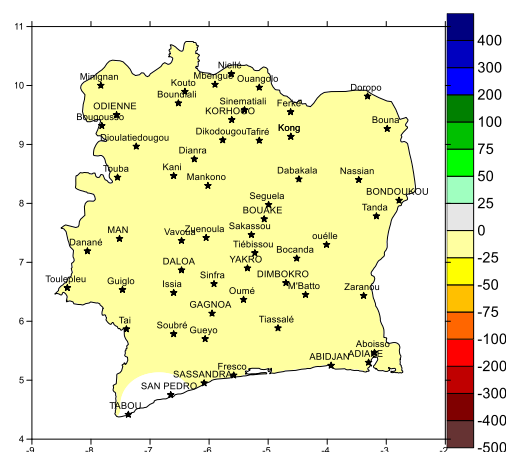
Fig2 : Ecarts entre la pluviométrie (mm) du 11 au 20 Janvier 2020 et du 11 au 20 Janvier de la normale (1981-2010)
