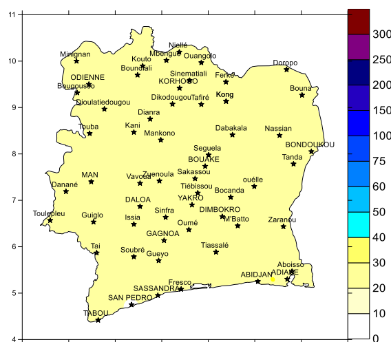
Fig. 4 : Ecart entre Cumuls pluviométriques du 1 au 20 Janvier 2020 et du 1 au 20 Janvier au de la normale (1981-2010)
