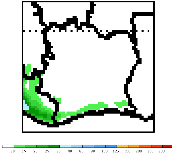
Fig.10: prévision de la pluviométrie du 23 au 30 Janvier 2020 (source : NOAA, climat Prédiction Center)
