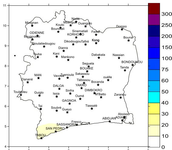
Fig. 3 : Cumul pluviométrique (mm) du 1 au 20 Janvier 2020
