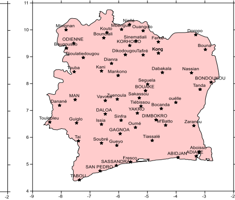
Fig 7 : ISBE des cultures annuelles en phase reproductive ou cultures pérennes
