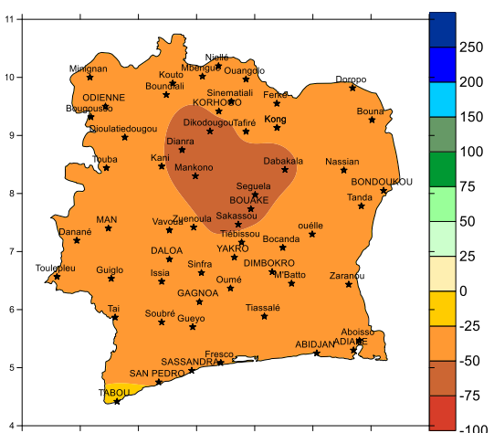
Fig. 9 : Bilan hydrique climatique (mm) du 1 au 10 Janvier 2020
